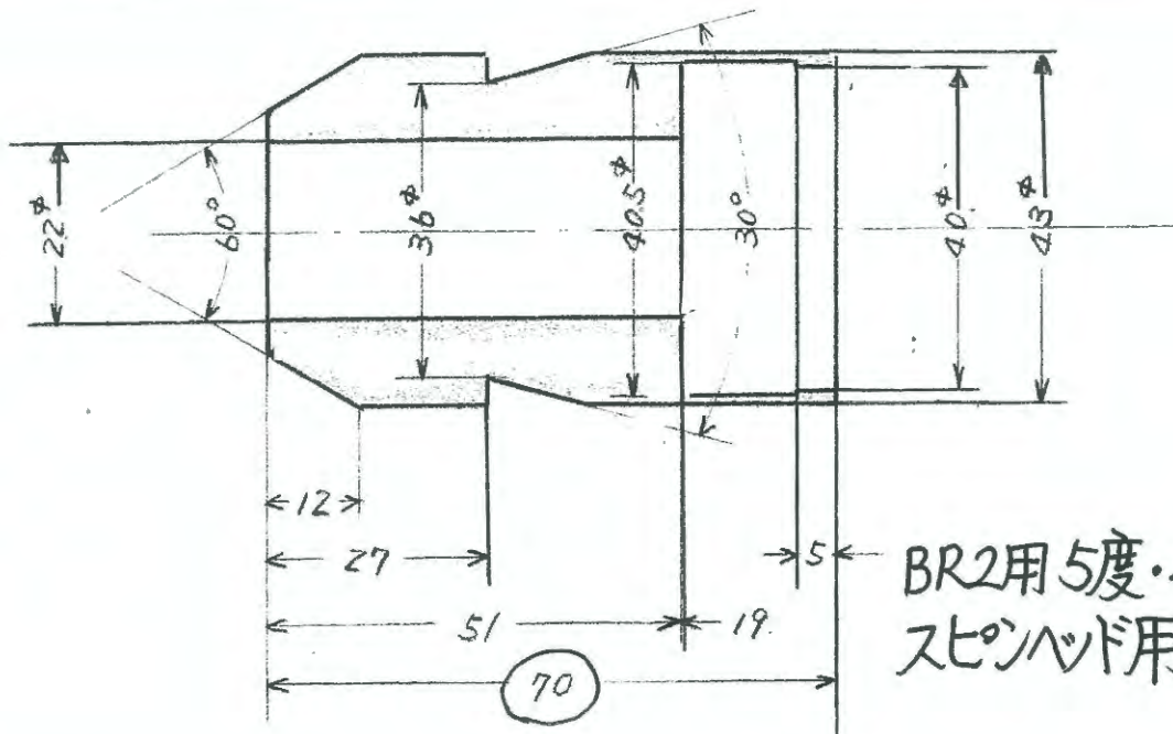
606877001 ベアリングホルダ-#2 (全長 70)
